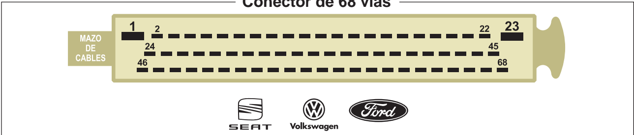
Conector de 68 vias
