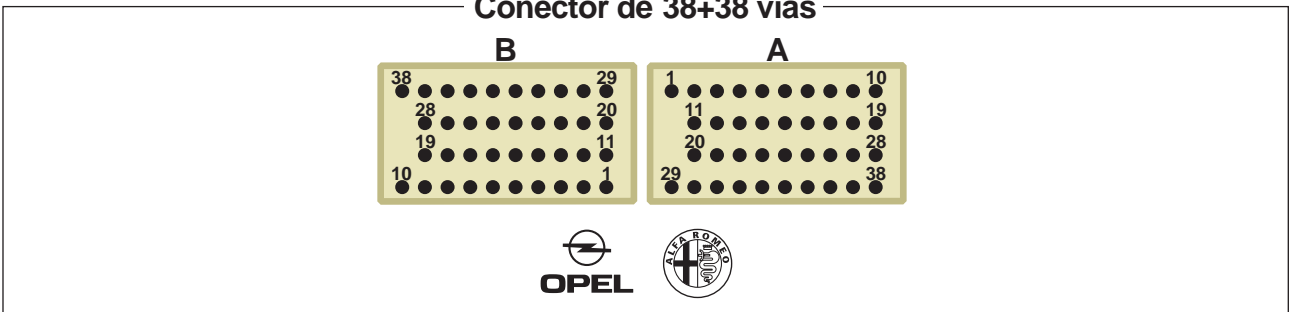
Conector de 38+38 vias
