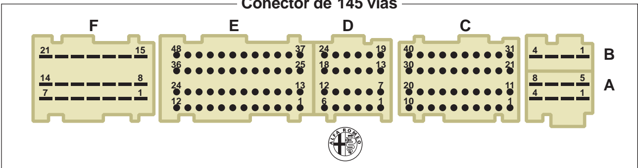
Conector de 145 vias
