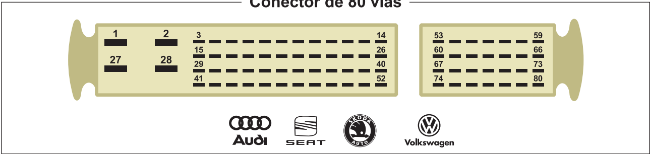
Conector de 80 vias
