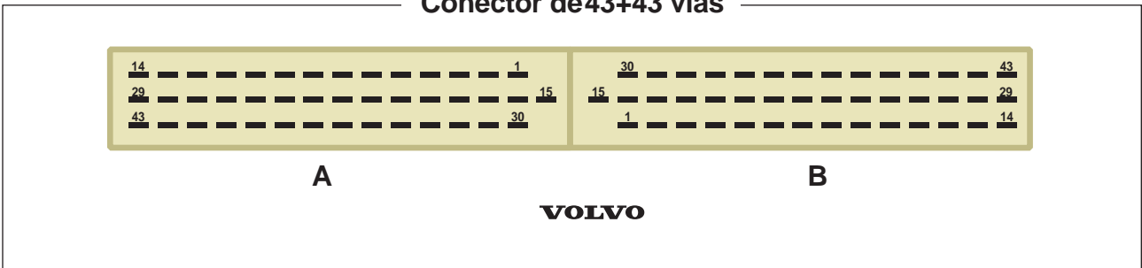
Conector de 43+43 vias
