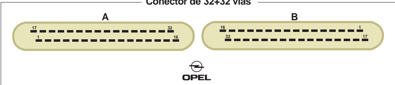
Conector de 32+32 vias
