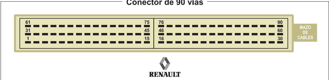
Conector de 90 vias
