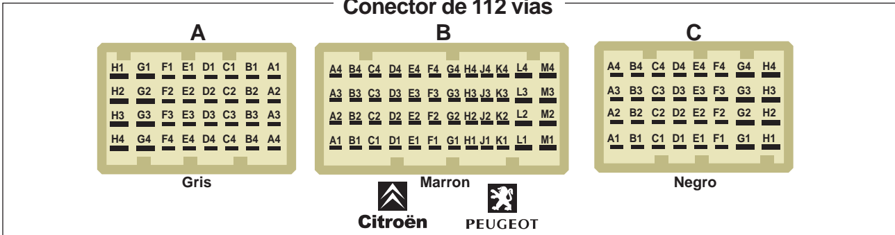
Conector de 112 vias
