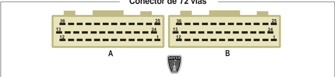
Conector de 72 vias
