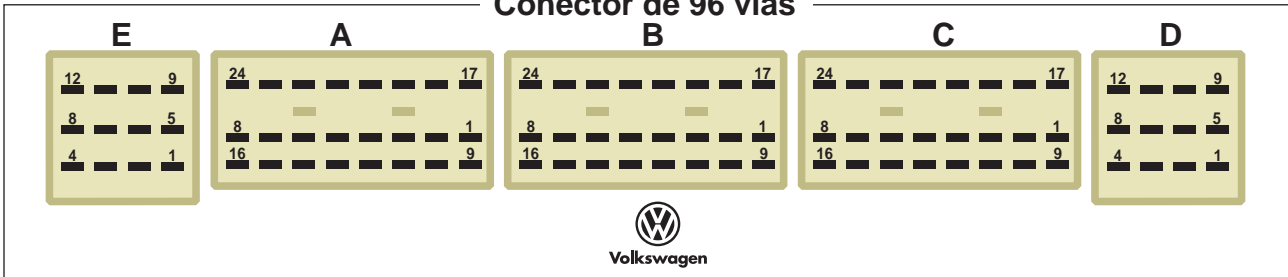
Conector de 96 vias
