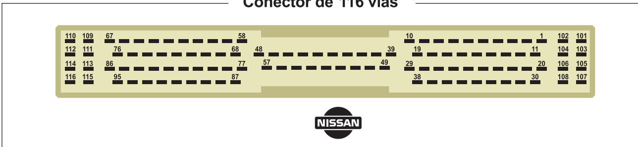
Conector de 116 vias
