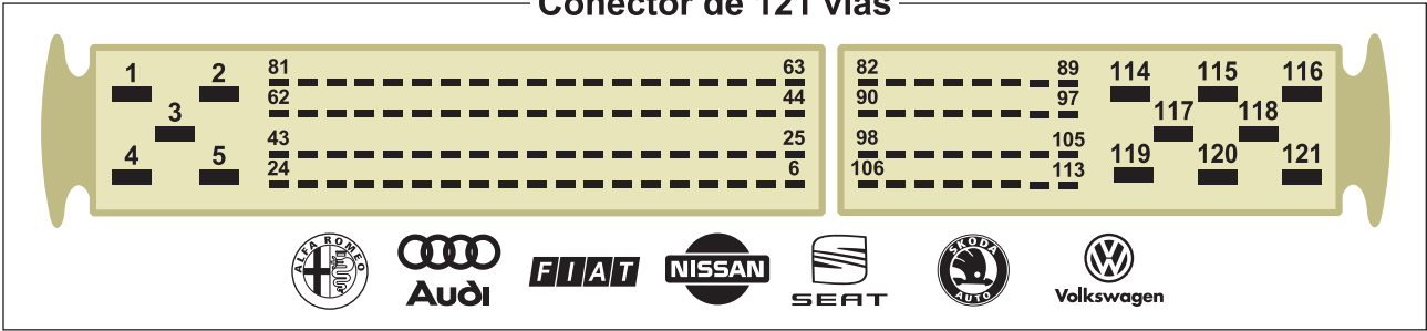
Conector de 64+64 vias
